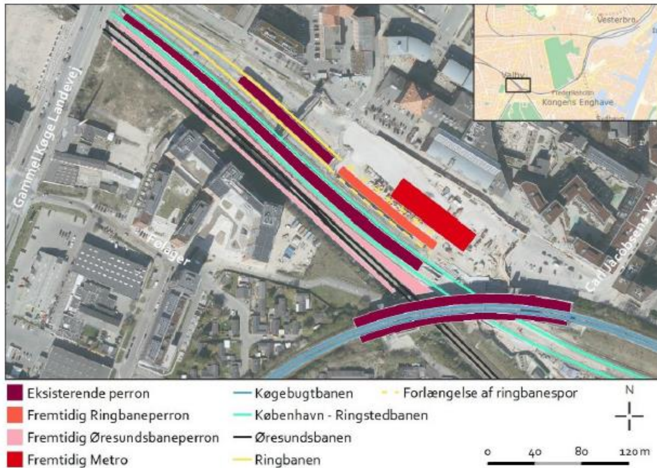
Figur 1-1: Oversigtskort af Ny Ellebjerg Station.
