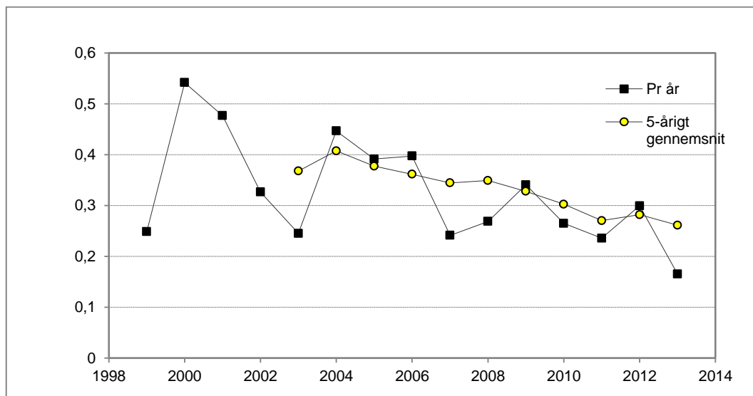
Figur 2: Væsentlige ulykker 1999 – 2013
